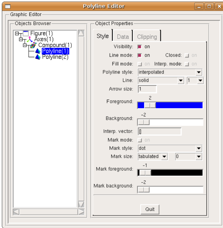
Рис. 4.26. Иерархия объектов в поле Object Browser
