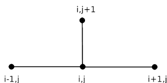
Рис. 12.2. Шаблон явной двухслойной разностной схемы
