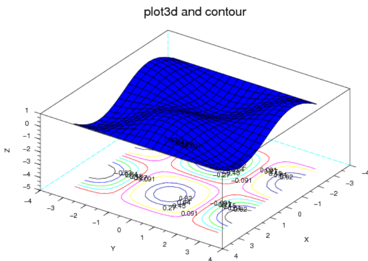
Рис. 5.20. График поверхности Z = \sin(x) \cdot \cos(y) и ее изолинии в одном окне
