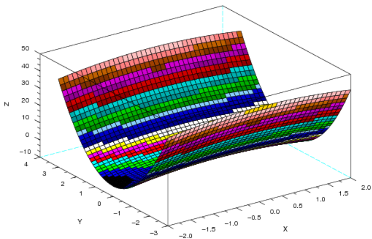
Рис. 5.14. График функции Z = 5y^2 - x^2 , построенный командой surf
