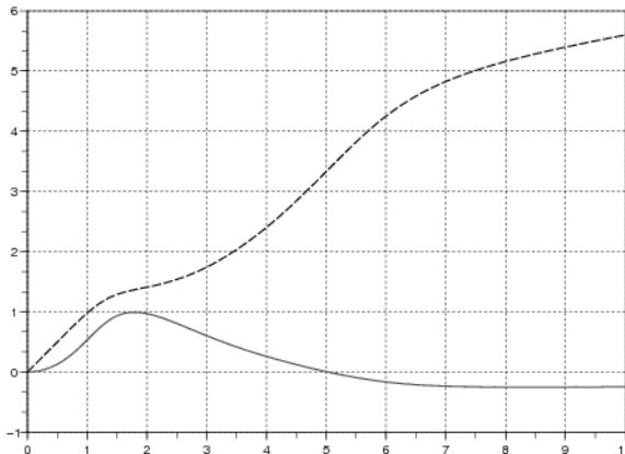
Рис. 8.2. Решение задачи 8.2
