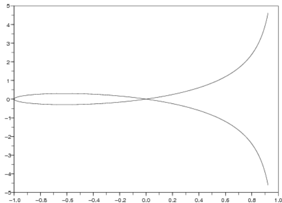
Рис. 4.22. График строфоиды
