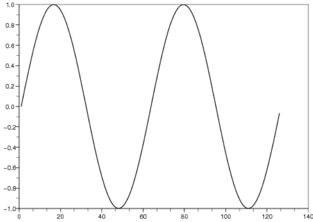
Рис. 4.8. График функции y = \sin(x)
