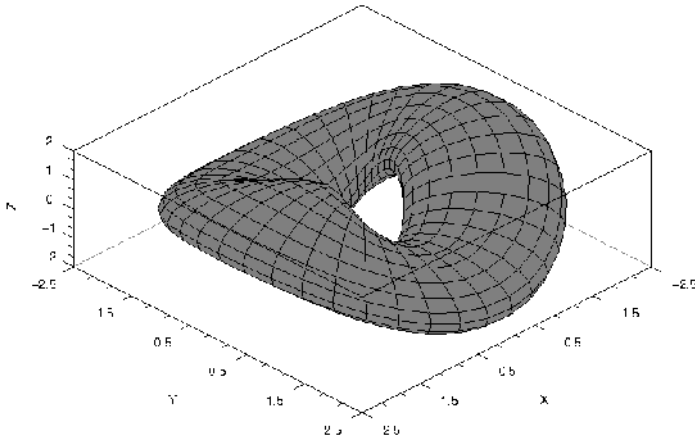
Рис. 5.10. Деформированный тор
