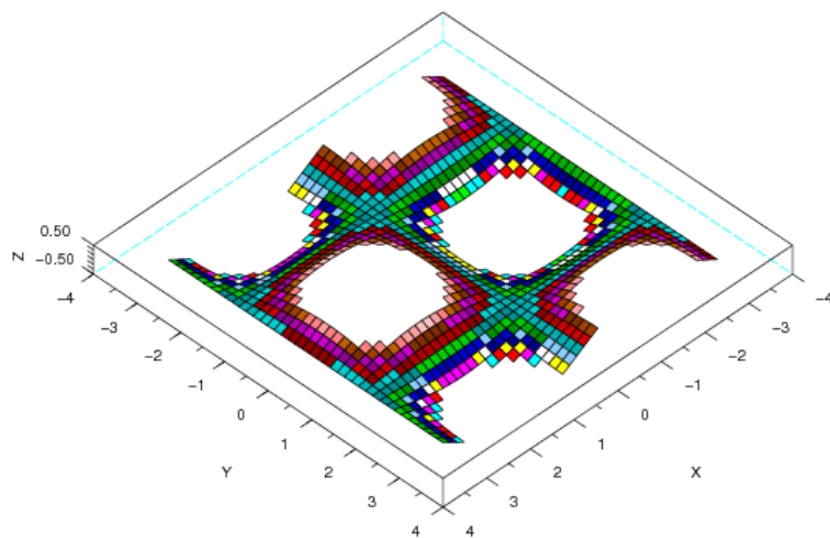
Рис. 5.23. Пример «вырезания» областей из трехмерного графика
