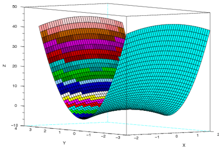
Рис. 5.12. График функции Z = 5y^2 - x^2
