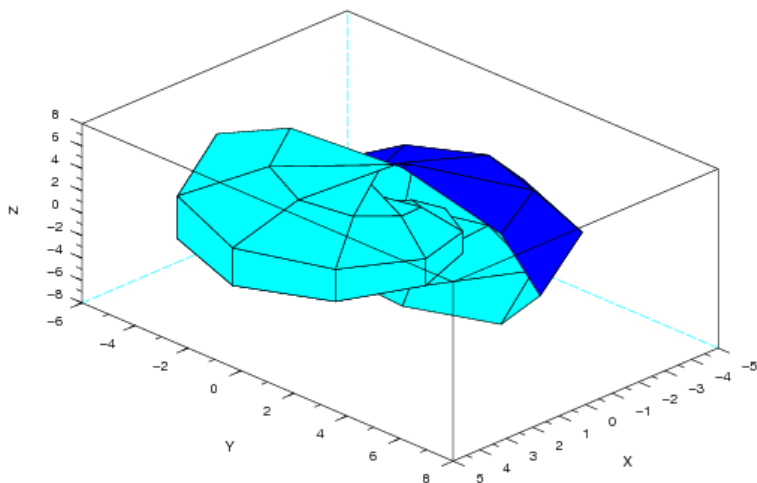
Рис. 5.13. График функции, построенный при помощи команды eval3df
