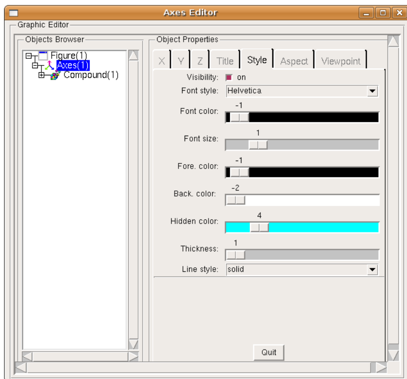
Рис. 4.37. Закладка Style окна форматирования осей Axes Editor
