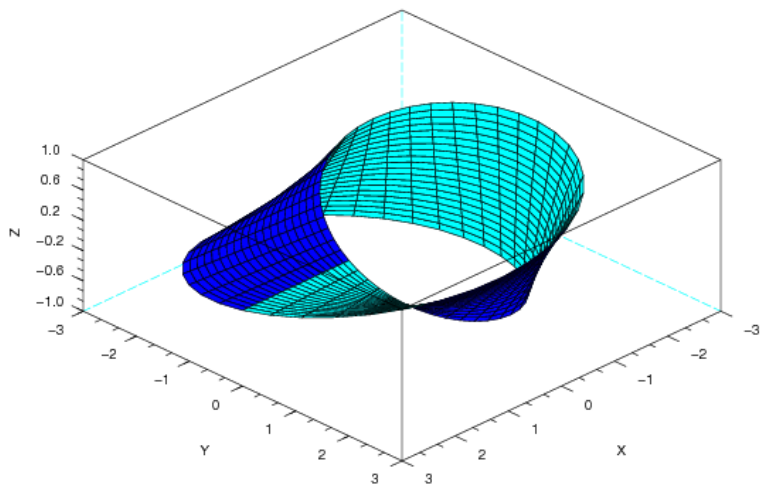
Рис. 5.26. Лента Мебиуса
