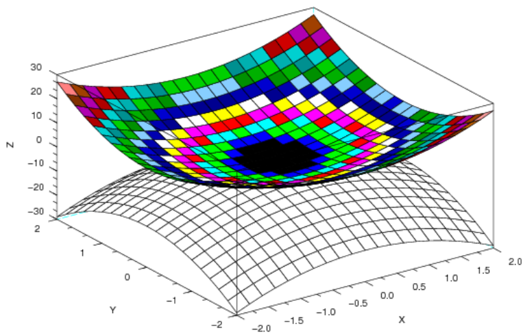
Рис. 5.16. График функции z(x, y) = \pm(3x^2 + 4y^2) - 1
