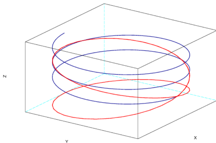
Рис. 5.18. Графики параметрических кривых, построенные функцией param3d1
