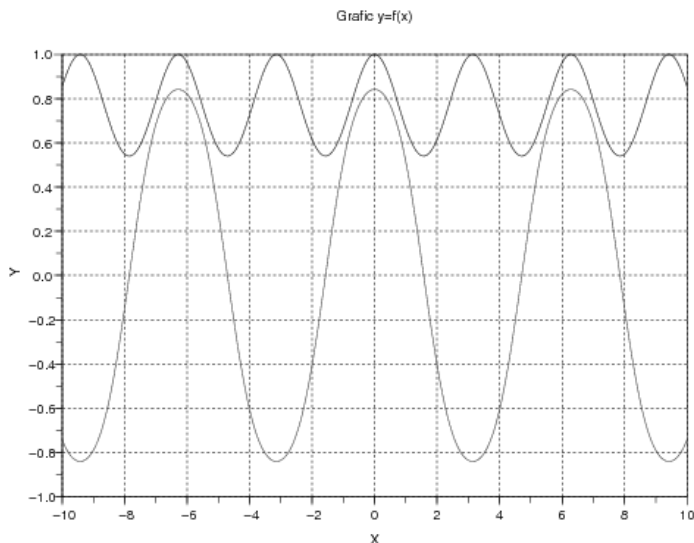
Рис. 4.12. Команда xtitle
