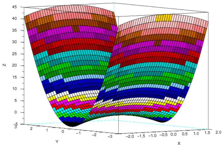
Рис. 5.15. График функции Z = 5y^2 - x^2 при отключенном режиме Cube scaling
