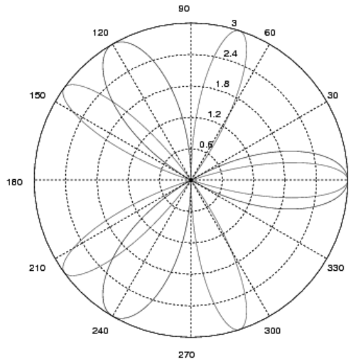
Рис. 4.21. Полярные графики функций \rho = 3 \cos(5\varphi) , \rho_1 = 3 \cos(3\varphi)
