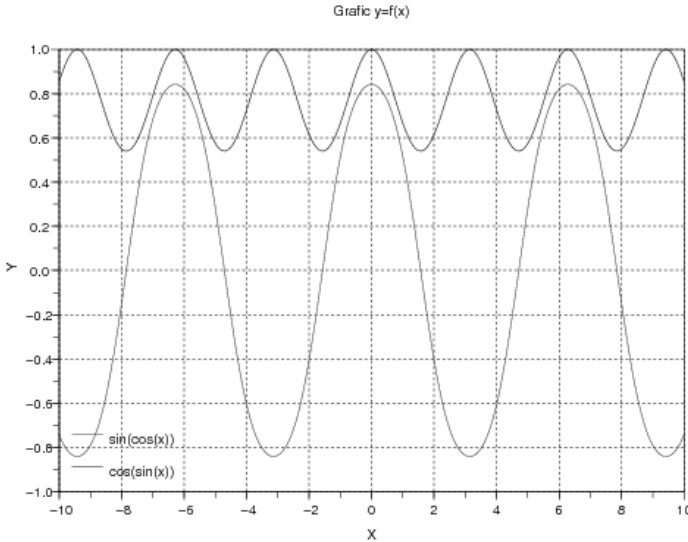
Рис. 4.13. Команда legend
