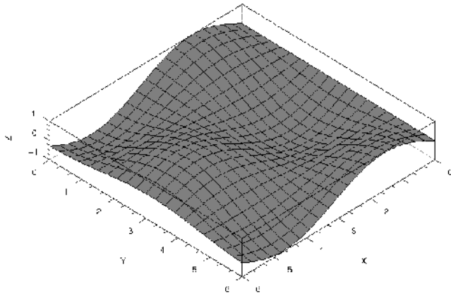
Рис. 5.1. График функции Z = \sin(t) \cdot \cos(t)
