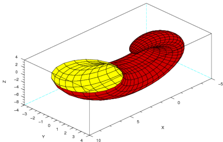
Рис. 5.25. Ракушкообразный график, построенный функцией plot3d2
