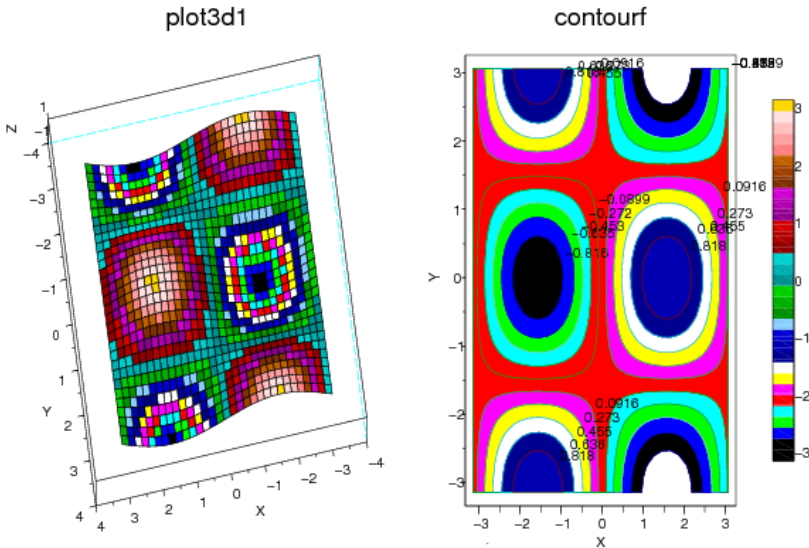
Рис. 5.22. График функции Z = \sin(x) \cdot \cos(y) , построенный функцией plot3d1 и contourf.
