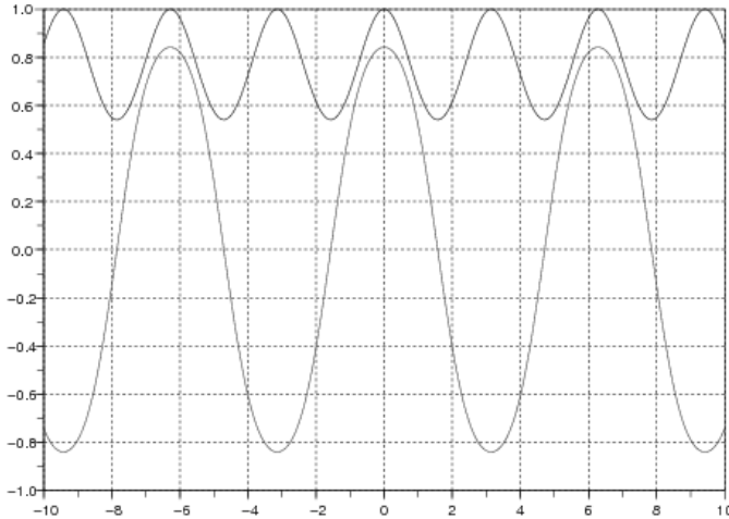
Рис. 4.11. Команда xgrid
