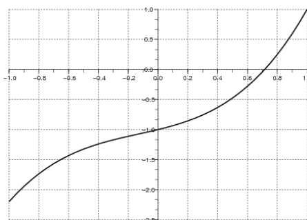
Рис. 6.2. Графическое решение задачи 6.2
