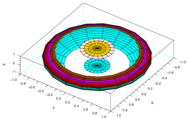
Рис. 5.24. График полый сферы
