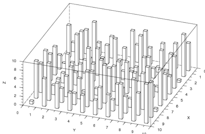
Рис. 5.8. Трехмерная гистограмма, построенная функцией hist3d
