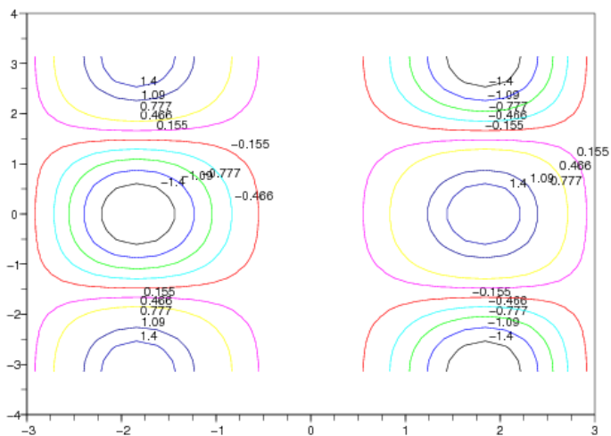
Рис. 5.19. Изолинии поверхности Z = x \cdot \sin(x)^2 \cdot \cos(y)
