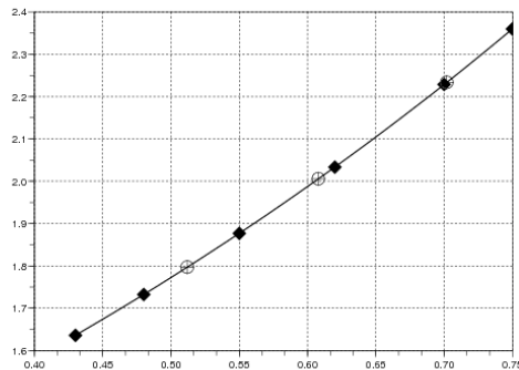
Рис. 11.5. Решение задачи 11.4
