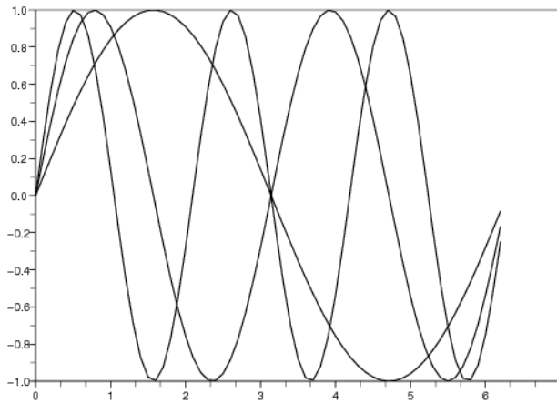
Рис. 4.9. Графики функций y = \sin(x) , y = \sin(2x) , y = \sin(3x)
