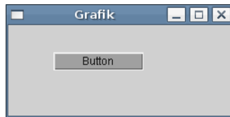
Рис. 10.6. Окно программы
